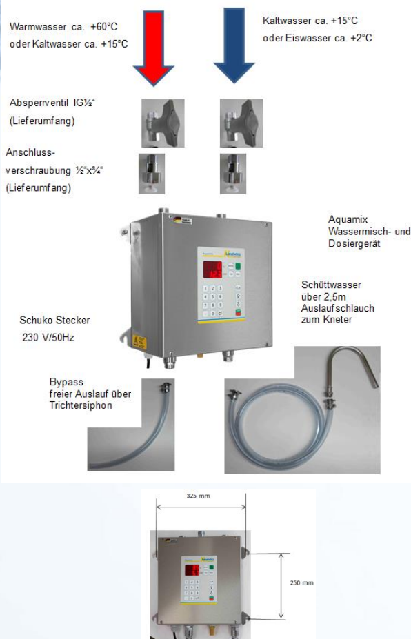
Anschluss-Schema
